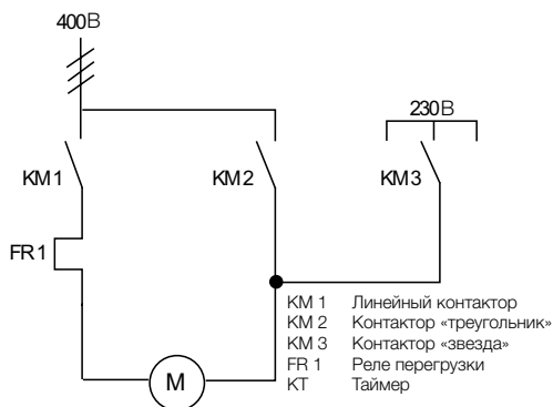
Пускатель со схемой соединения звезда/треугольник с контакторами и реле перегрузки
