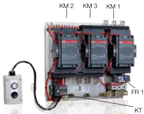
Пускатель со схемой соединения звезда/треугольник с контакторами и реле перегрузки
