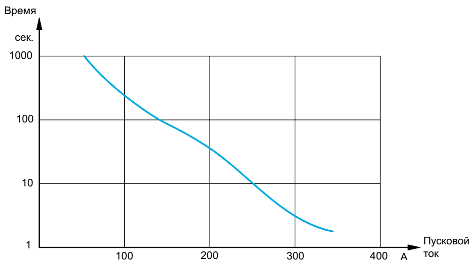
Примерный график пусковой способности для устройства плавного пуска
