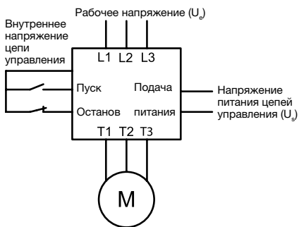
Устройства плавного пуска с внутренним напряжением цепи управления
